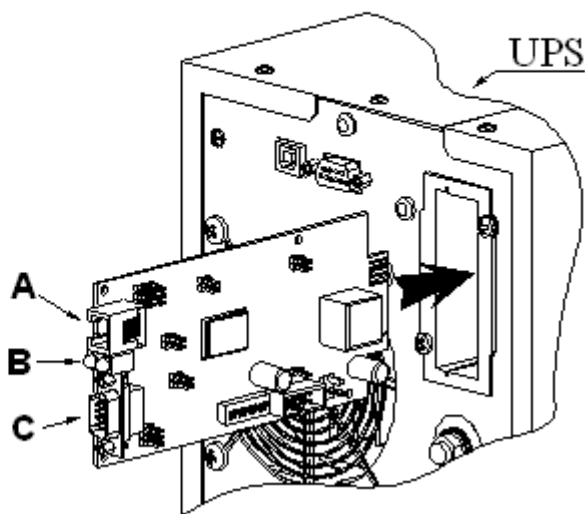
MultiCOM 302
